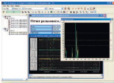
Отчет рельсового дефектоскопа УДС2-73
